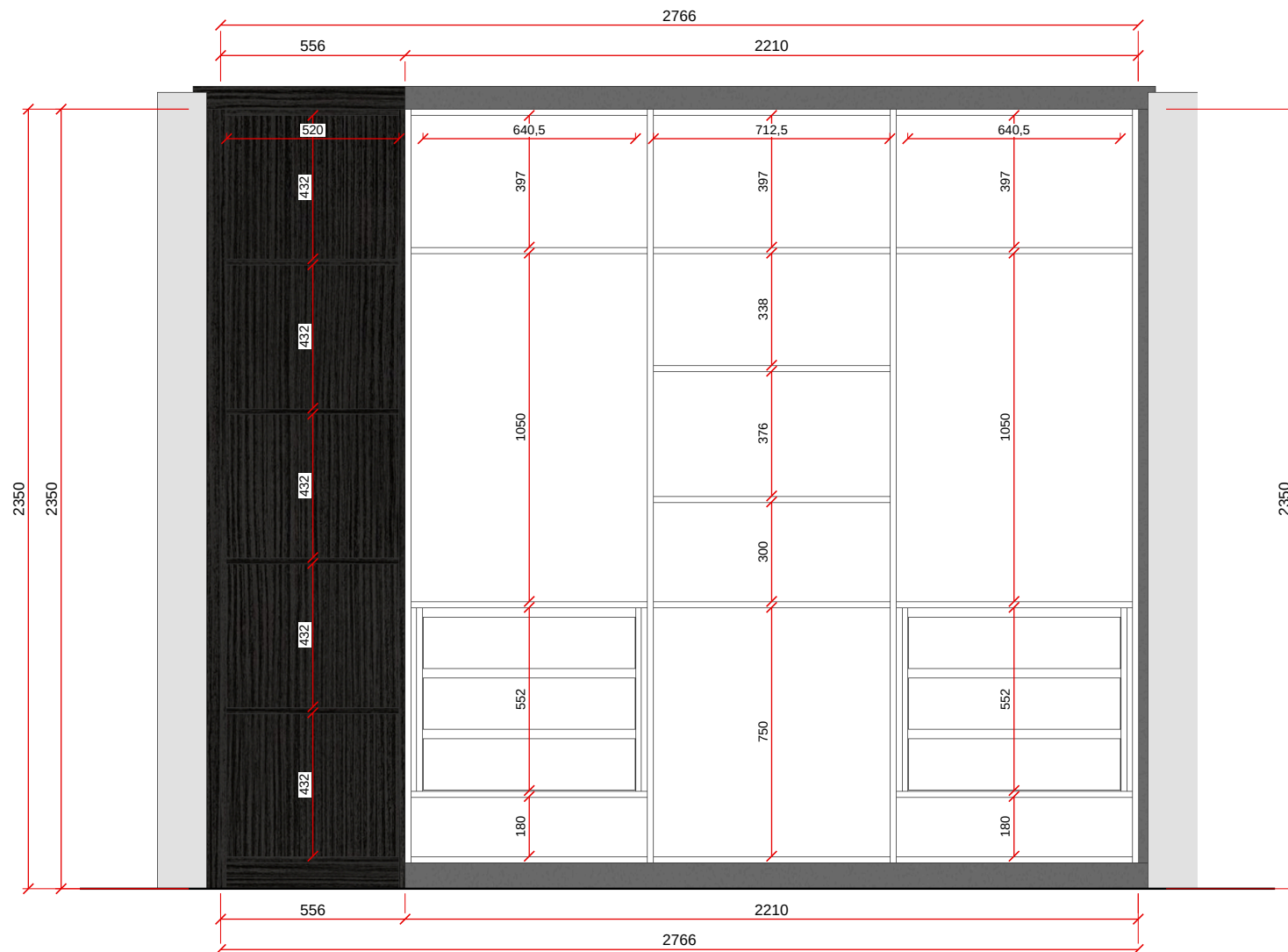
VISTA A - ESC. 1:20
